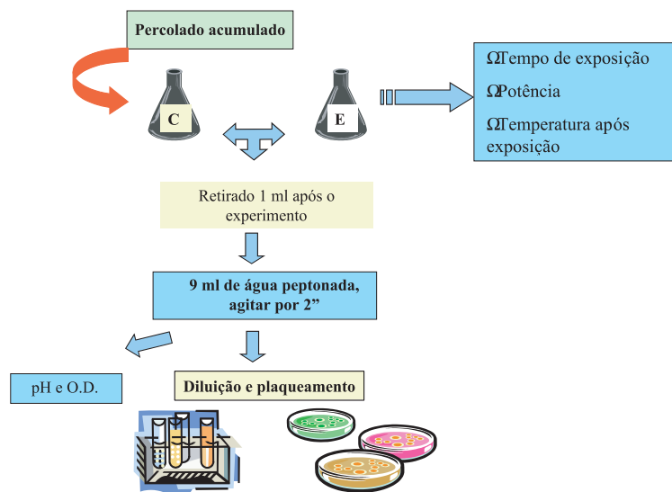
Figura 3.9 – Procedimento de desinfecção com o destrutor de células
