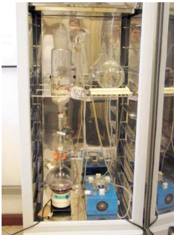
Figura 3.4 – Foto do reator em funcionamento
