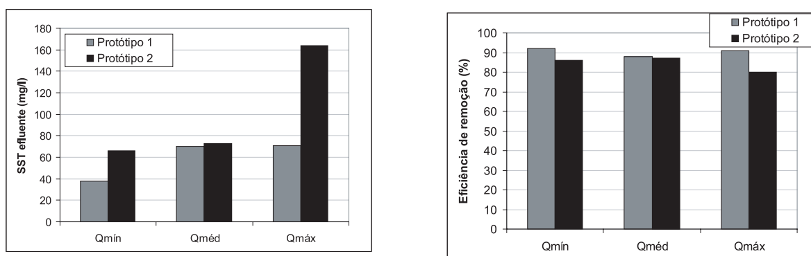
Figura 6.6 – Concentração média do efluente e eficiência média de remoção de SST – Fase 2
