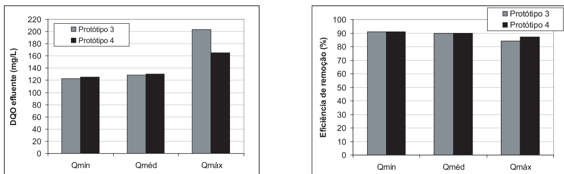
Figura 6.4 – Concentração média do efluente e eficiência média de remoção de DQO– Etapa 2
