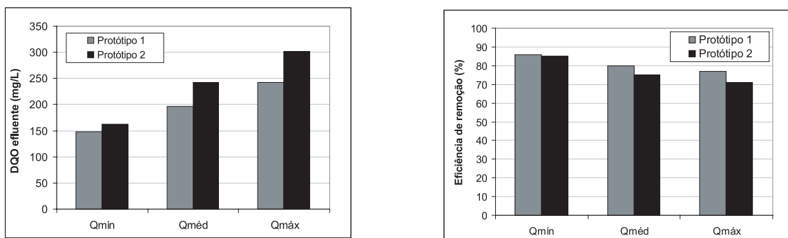
Figura 6.3 – Concentração média do efluente e eficiência média de remoção de DQO – Fase 3
