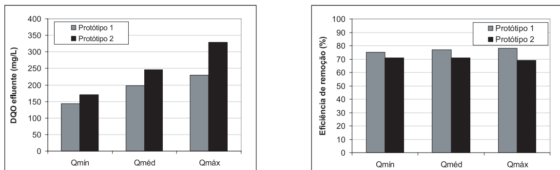
Figura 6.2 – Concentração média do efluente e eficiência média de remoção de DQO – Fase 2
