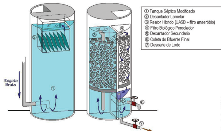
Figura 5.2 – Sistema compacto de tratamento de esgotos – SICOTE (Configurações 1 e 2)
