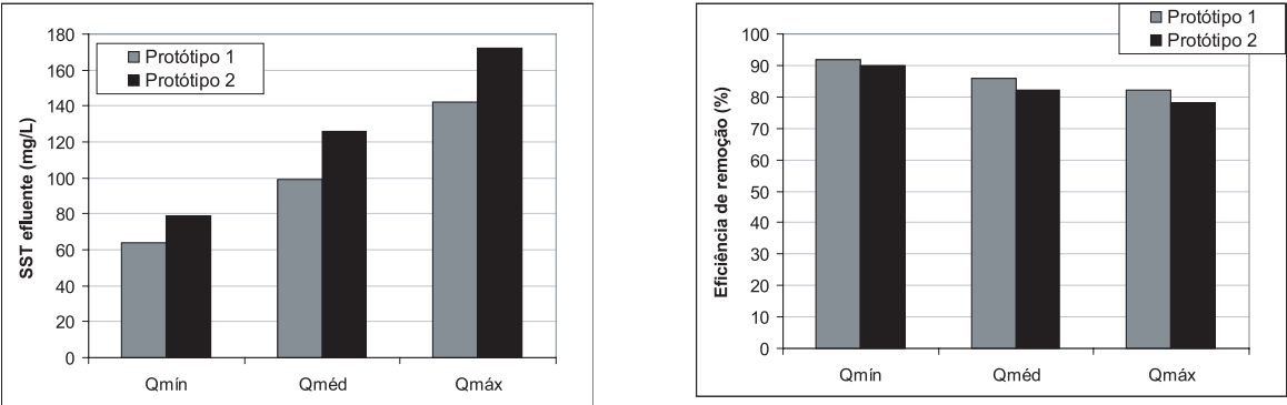
Figura 6.7 – Concentração média do efluente e eficiência média de remoção de SST – Fase 3
