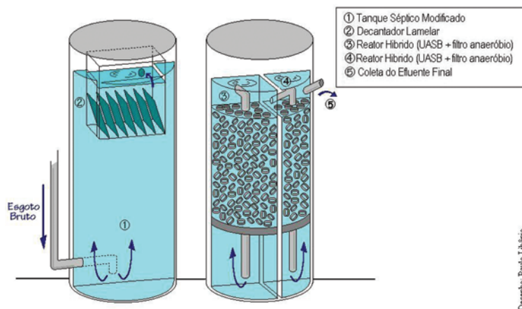
Figura 5.3– Sistema compacto de tratamento de esgotos – SICOTE (Configurações 3 e 4)
