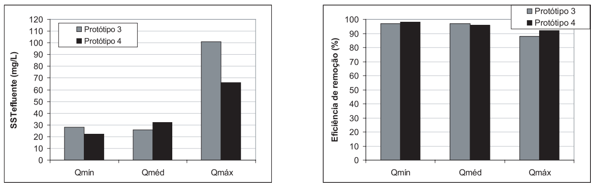
Figura 6.8 – Concentração média do efluente e eficiência média de remoção de SST– Etapa 2
