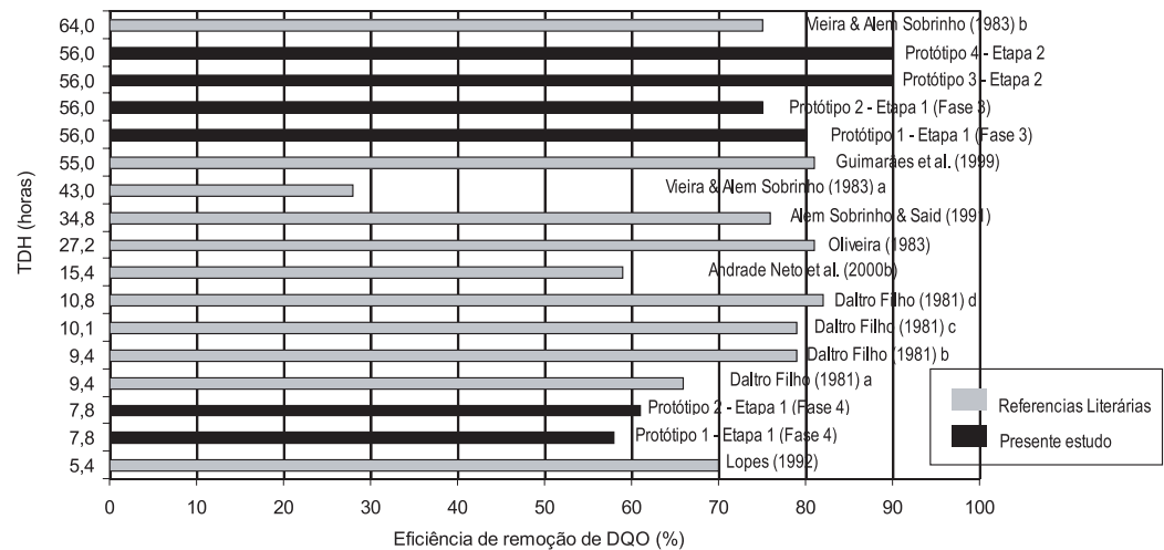
Figura 6.9 – Gráfico comparativo entre os diversos resultados de eficiência de remoção de DQO
